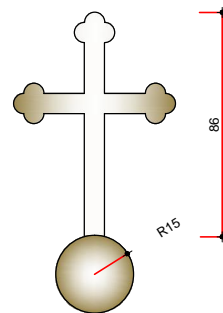
ESFERA (E-2); CRUZ (C-3) Esc. 1/12.5
