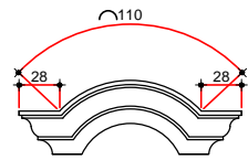
MOLDURA (M-2)a Esc. 1/25
