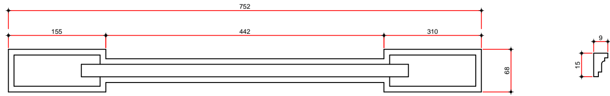
MOLDURA (M-1) Esc. 1/25
