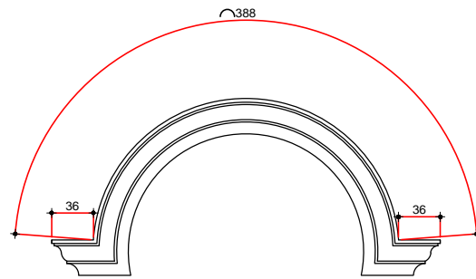
MOLDURA (M-2b) Esc. 1/25
